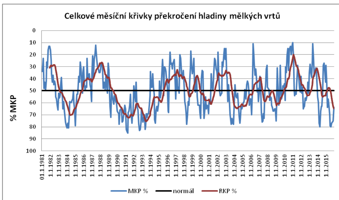
Obr. 8 Normalizované odchylky (zařazení měsíční křivky překročení – MKP) hladiny mělkých vrtů za období 1981–2015 s ročním klouzavým průměrem (RKP), zdroj: ČHMÚ
